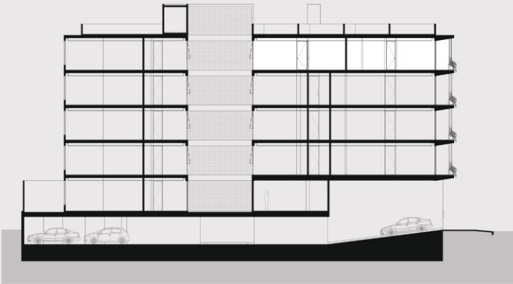
CORTE ESQUEMÁTICO
