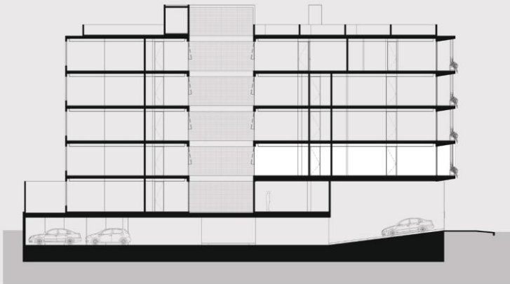
CORTE ESQUEMÁTICO
