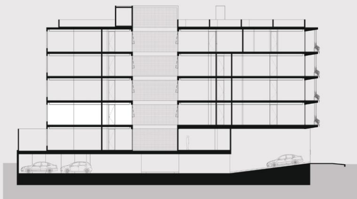
CORTE ESQUEMÁTICO
