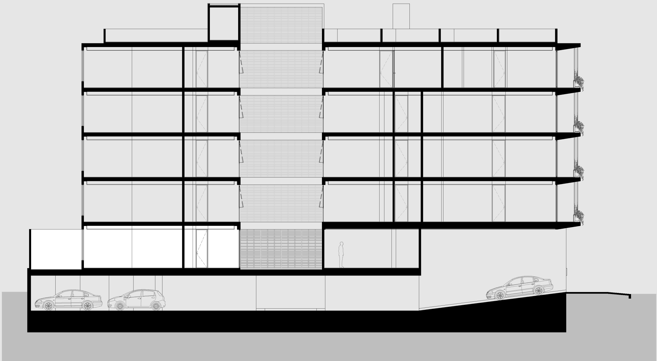
CORTE ESQUEMÁTICO
